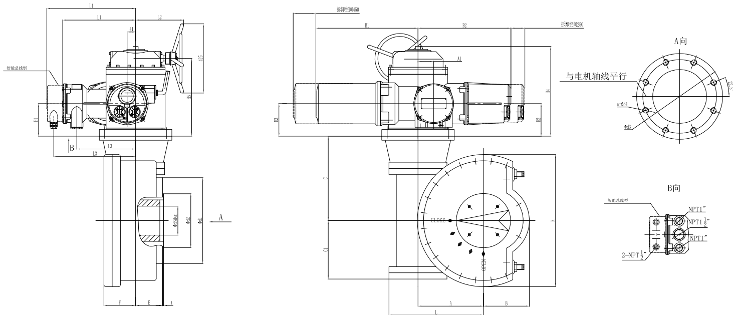
IMC100~300带HJBC系列外形及连接尺寸
